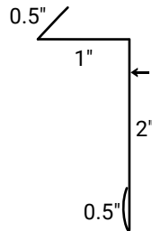
Reglet Flashing
