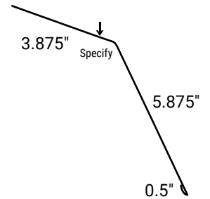
Gambrel
